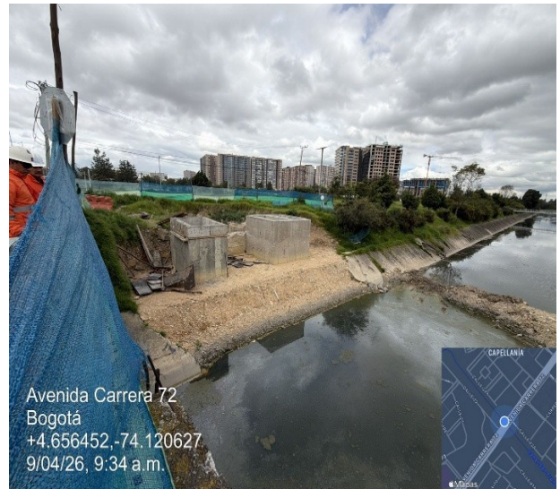
Fotografía No. 8. Vista lateral, cajas de inspección costado sur y lozas a renovar canal San Francisco.
