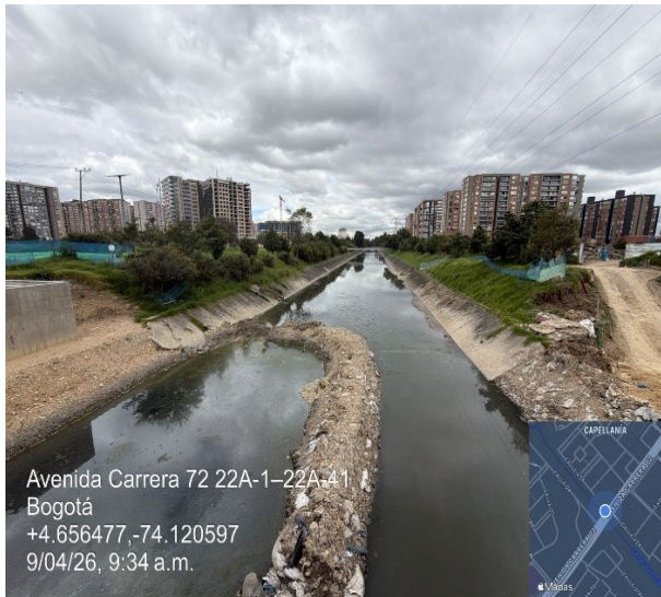
Fotografía No. 7. Vista frontal cauce canal san Francisco, lozas costado norte y sur a renovar y desvío temporal con bolsacreto en mal estado.
